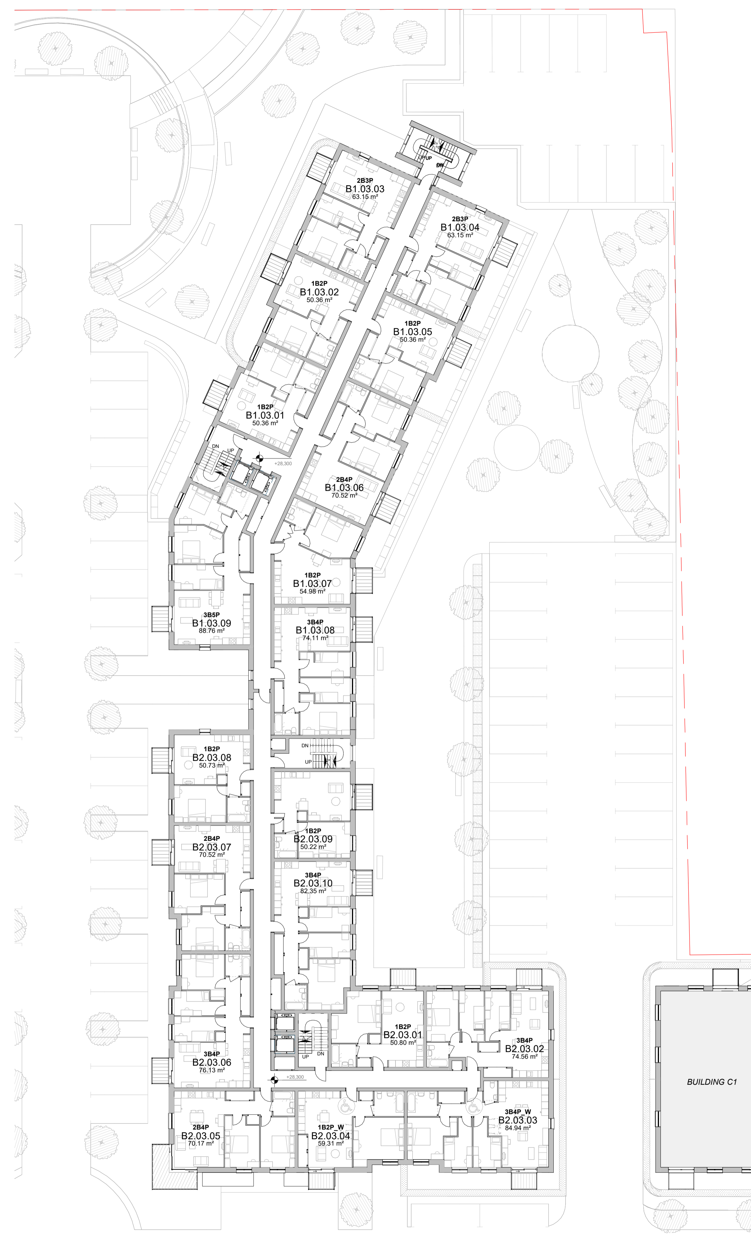
2 Level 3 +28.300 AOD 1:200
